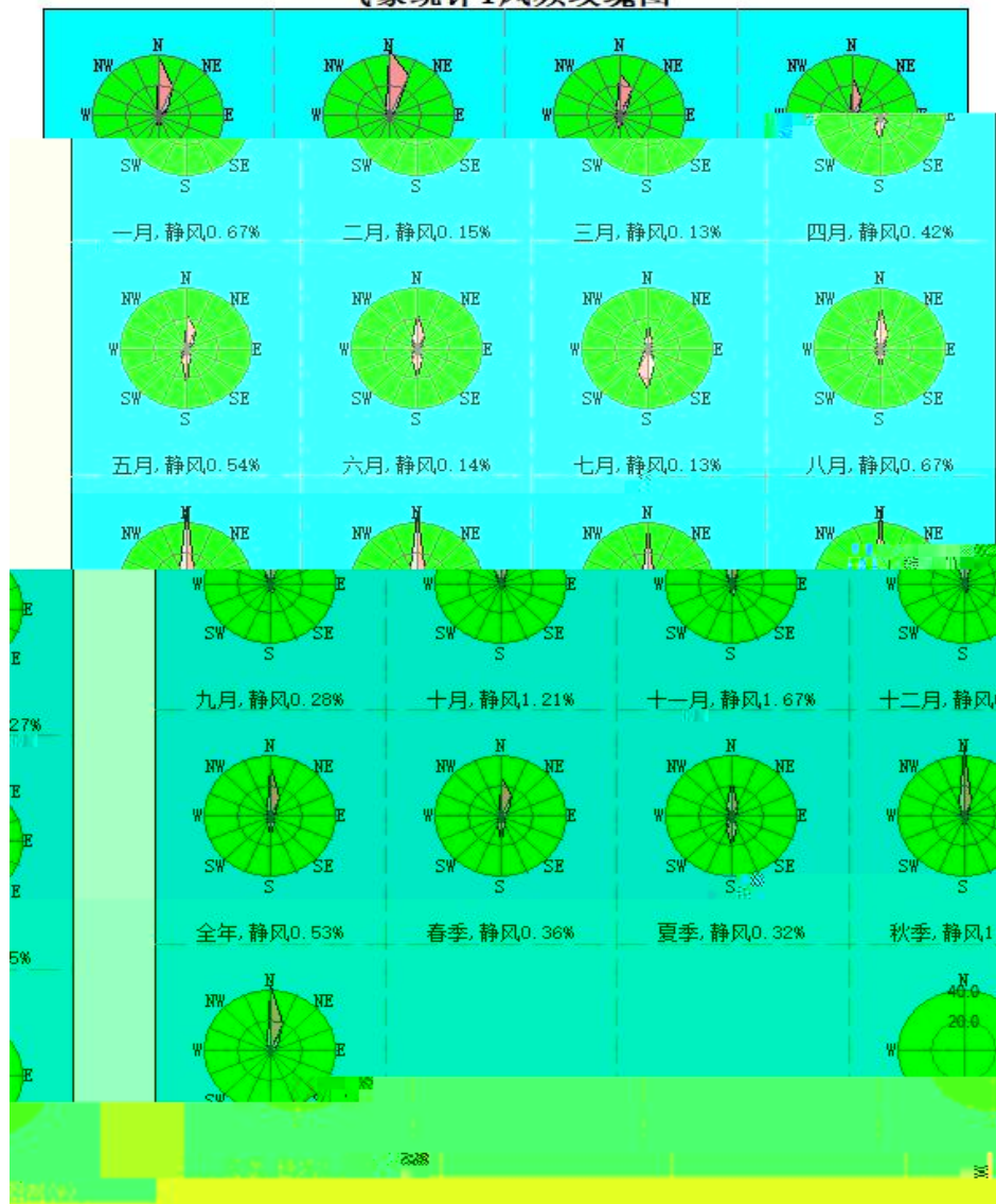
气象统计1风频玫瑰图
